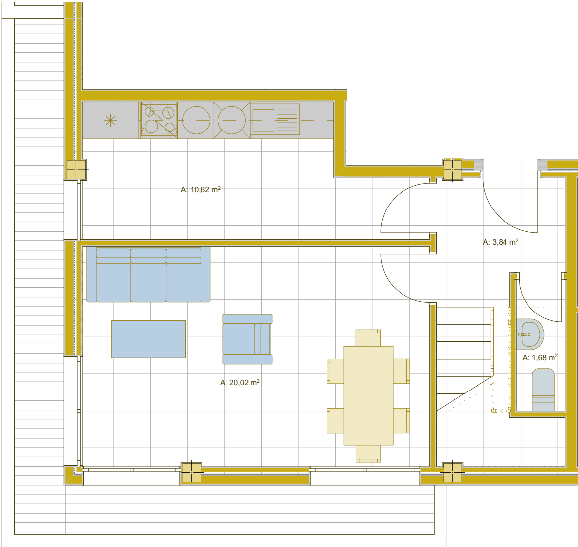
PLANTA PRIMERA
