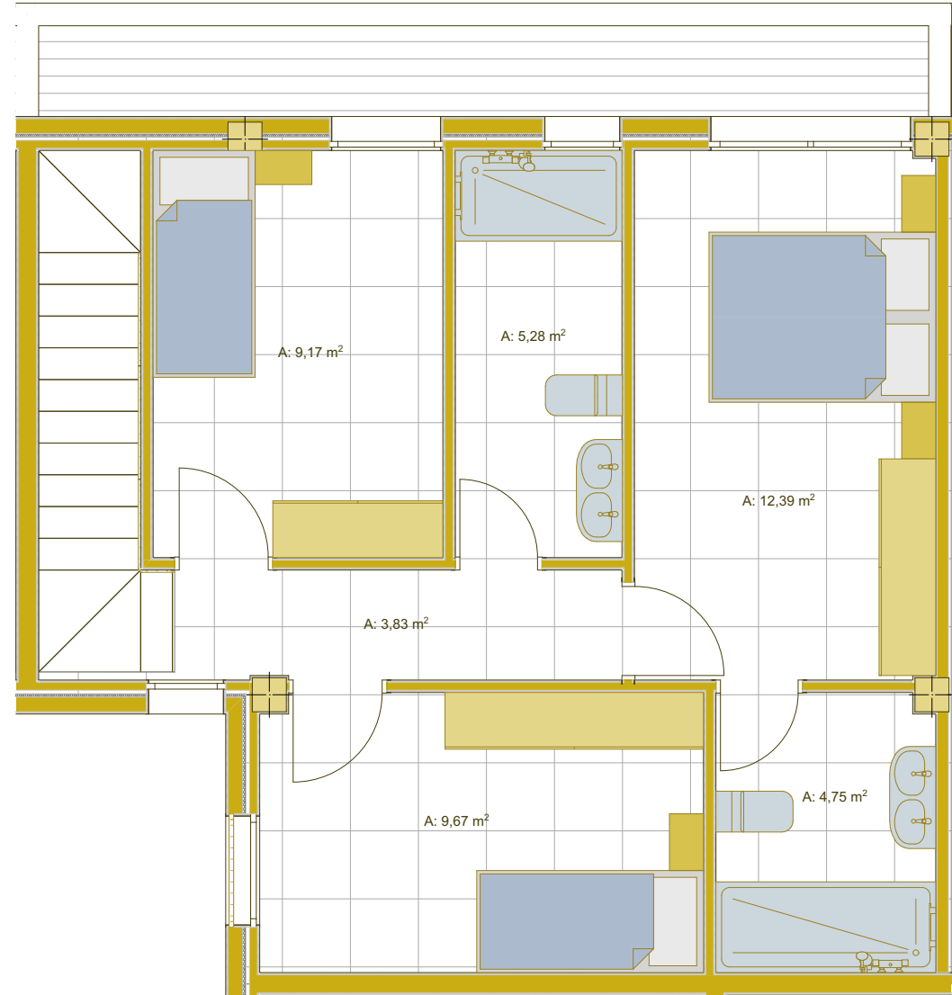
PLANTA SEGUNDA
