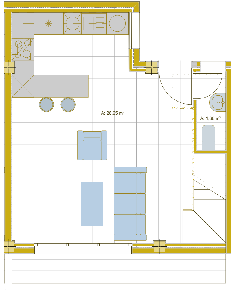
PLANTA PRIMERA
