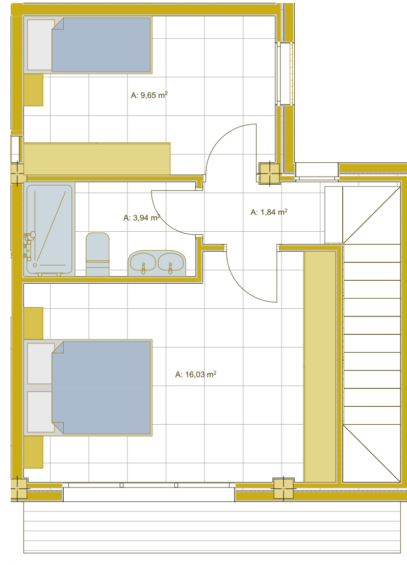
PLANTA SEGUNDA
