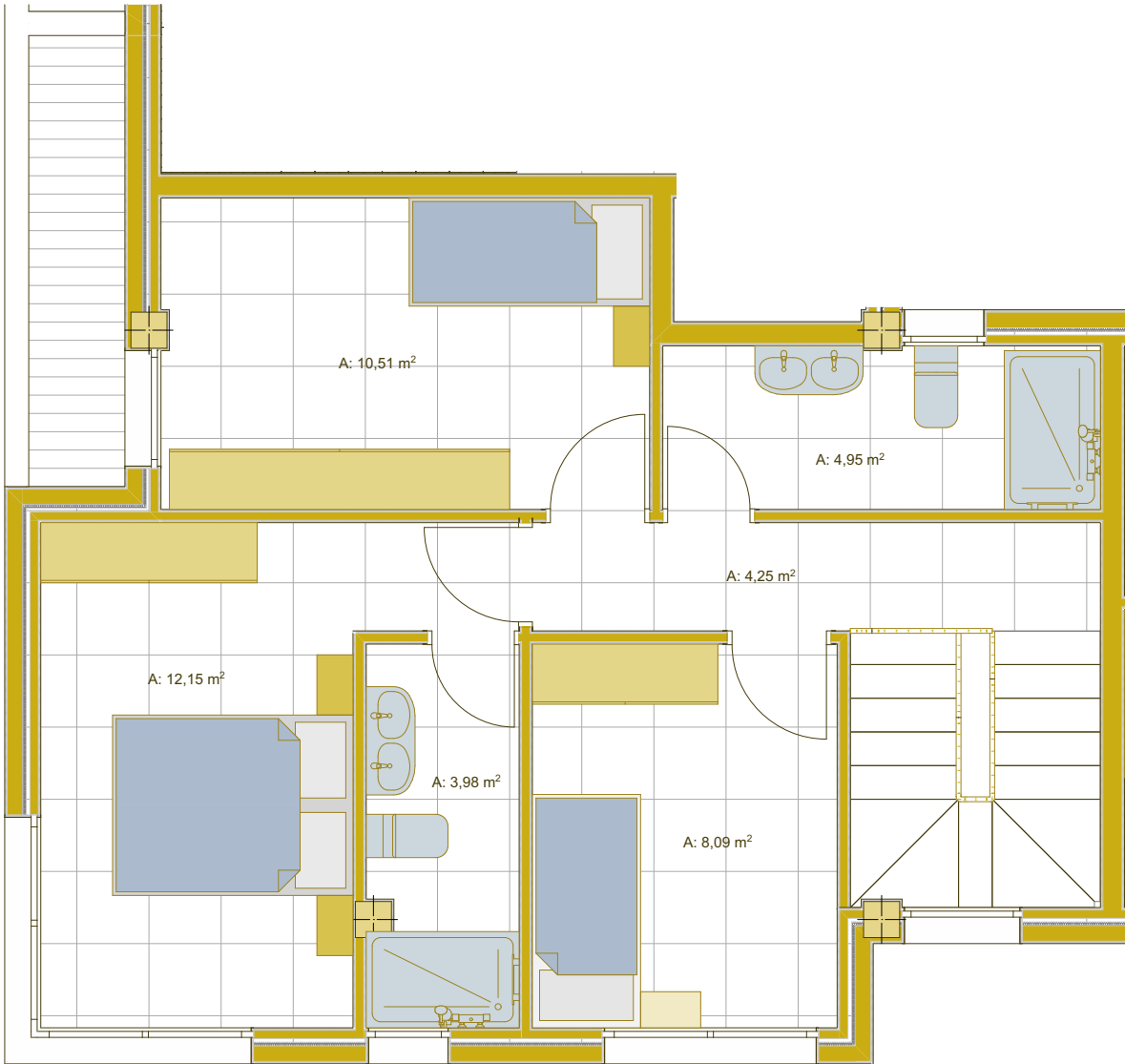
PLANTA SEGUNDA
