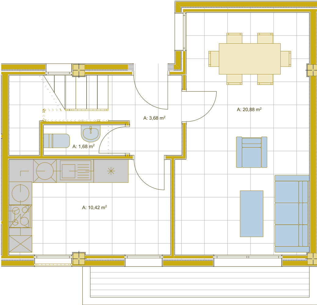
PLANTA PRIMERA
