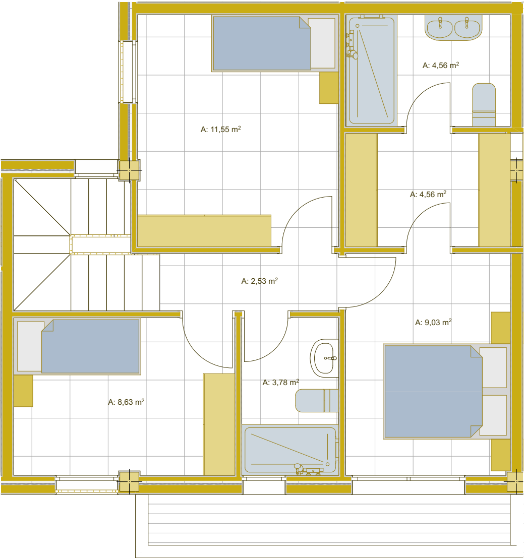
PLANTA SEGUNDA
