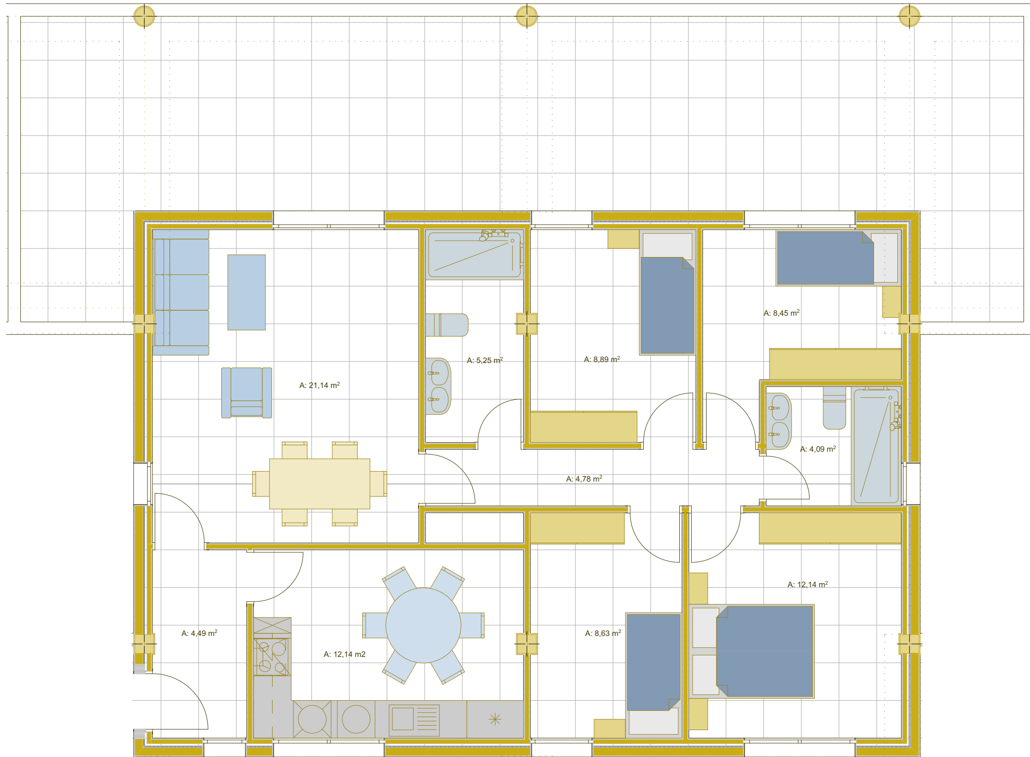
PLANTA ATICO
